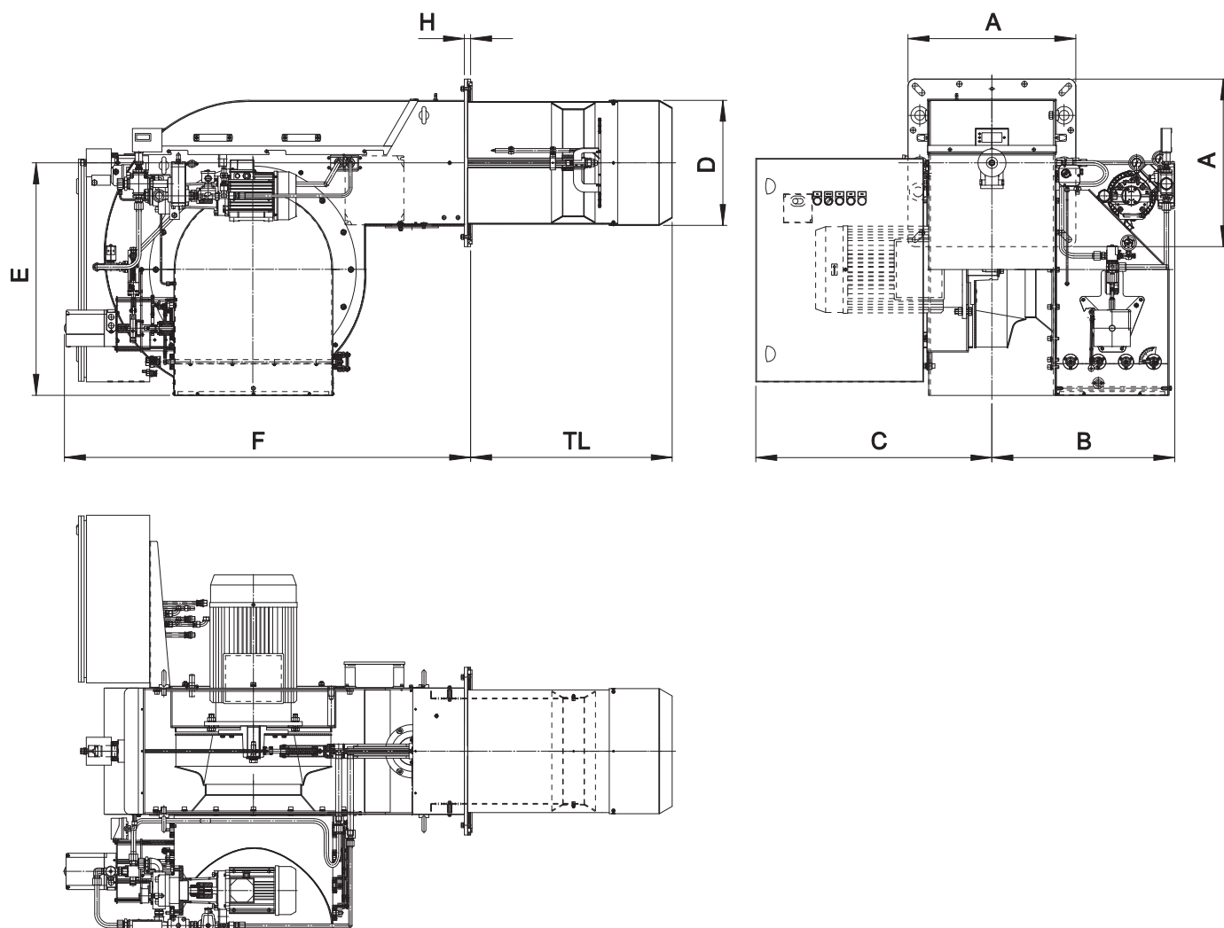
Fig. 6 Burner dimensions
