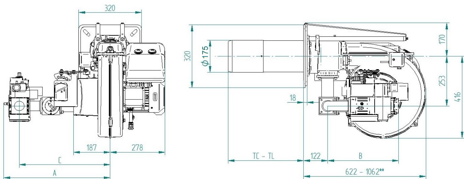
Fig. 3 Dimensions
