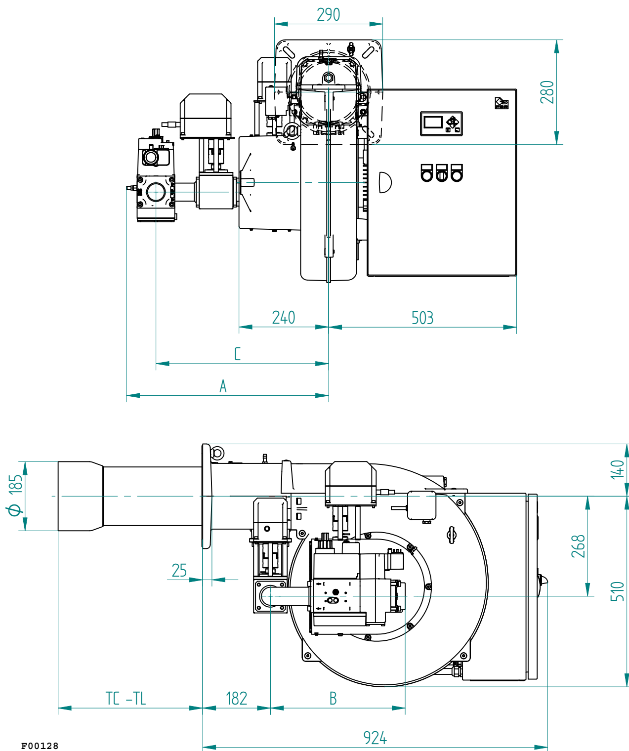
Fig. 4 Dimensions
