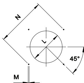
Fig. 4 Фланец для установки горелки
