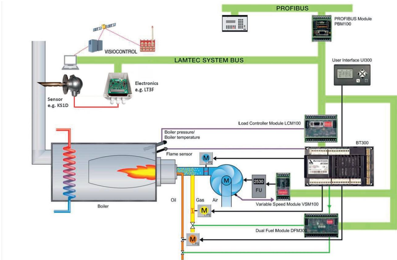
Fig. 5 Control box Lamtec BT3
