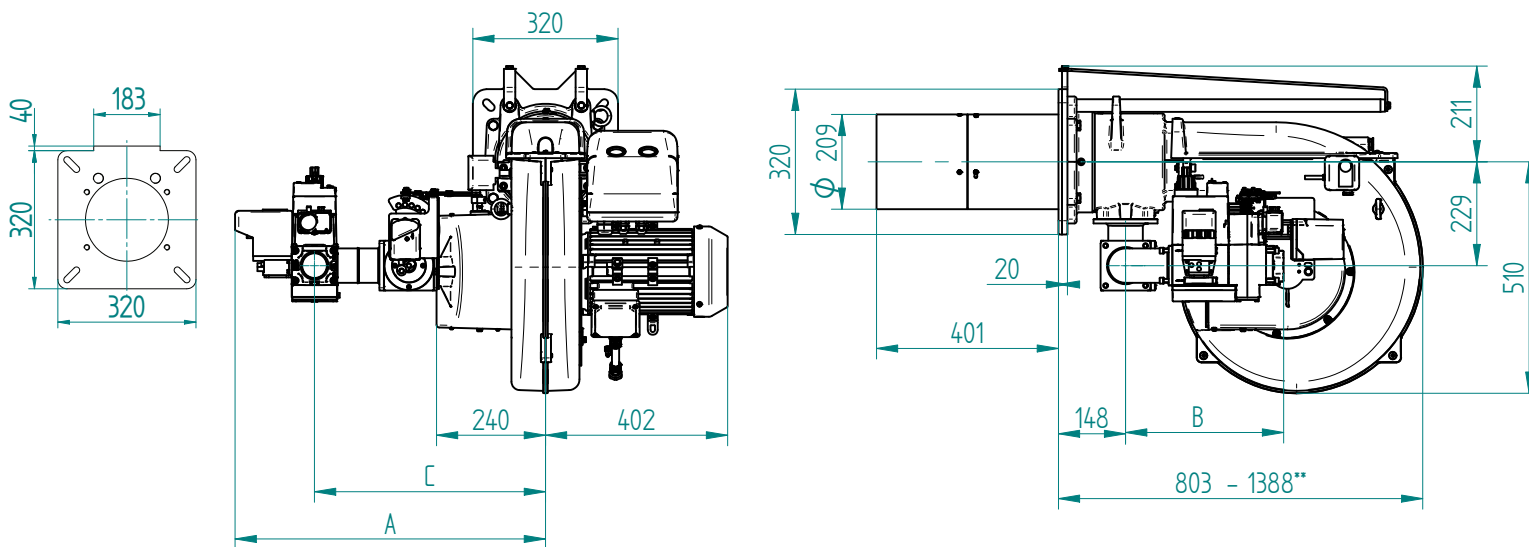
Fig. Dimensions GAS P160/MCE
