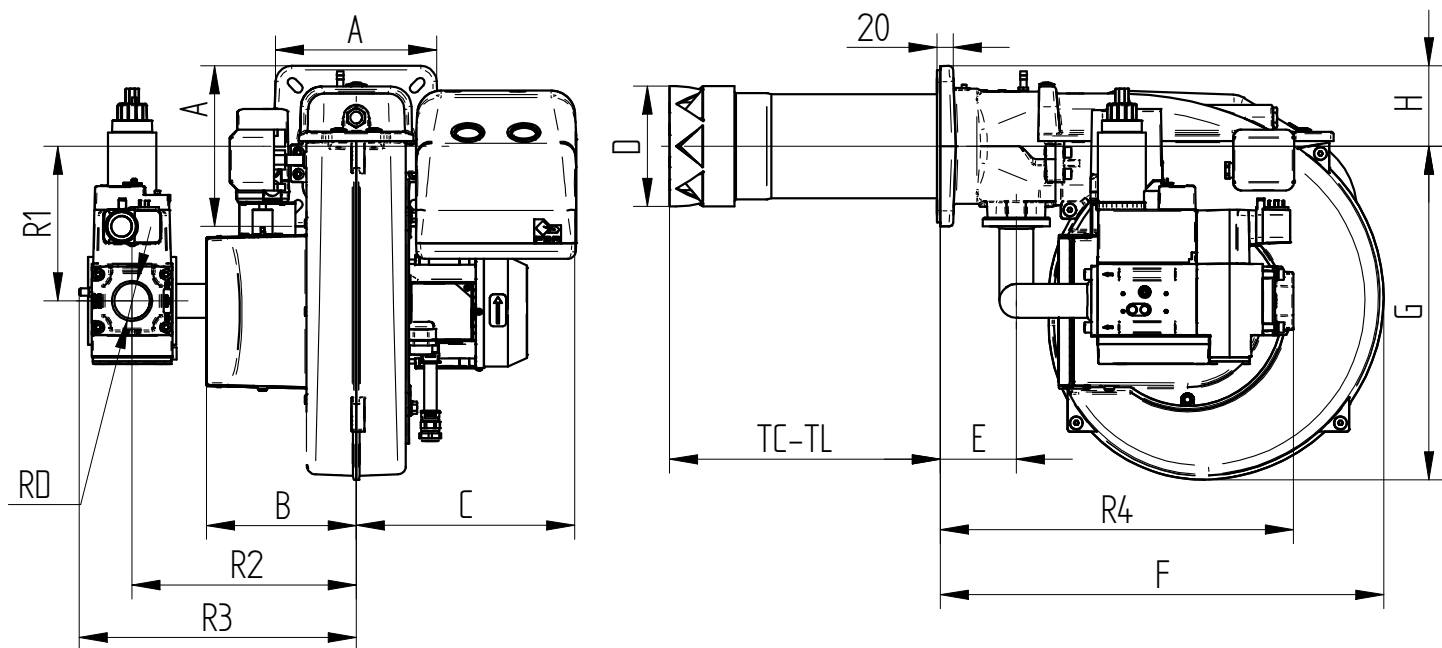
Fig. 2 РАЗМЕРЫ
