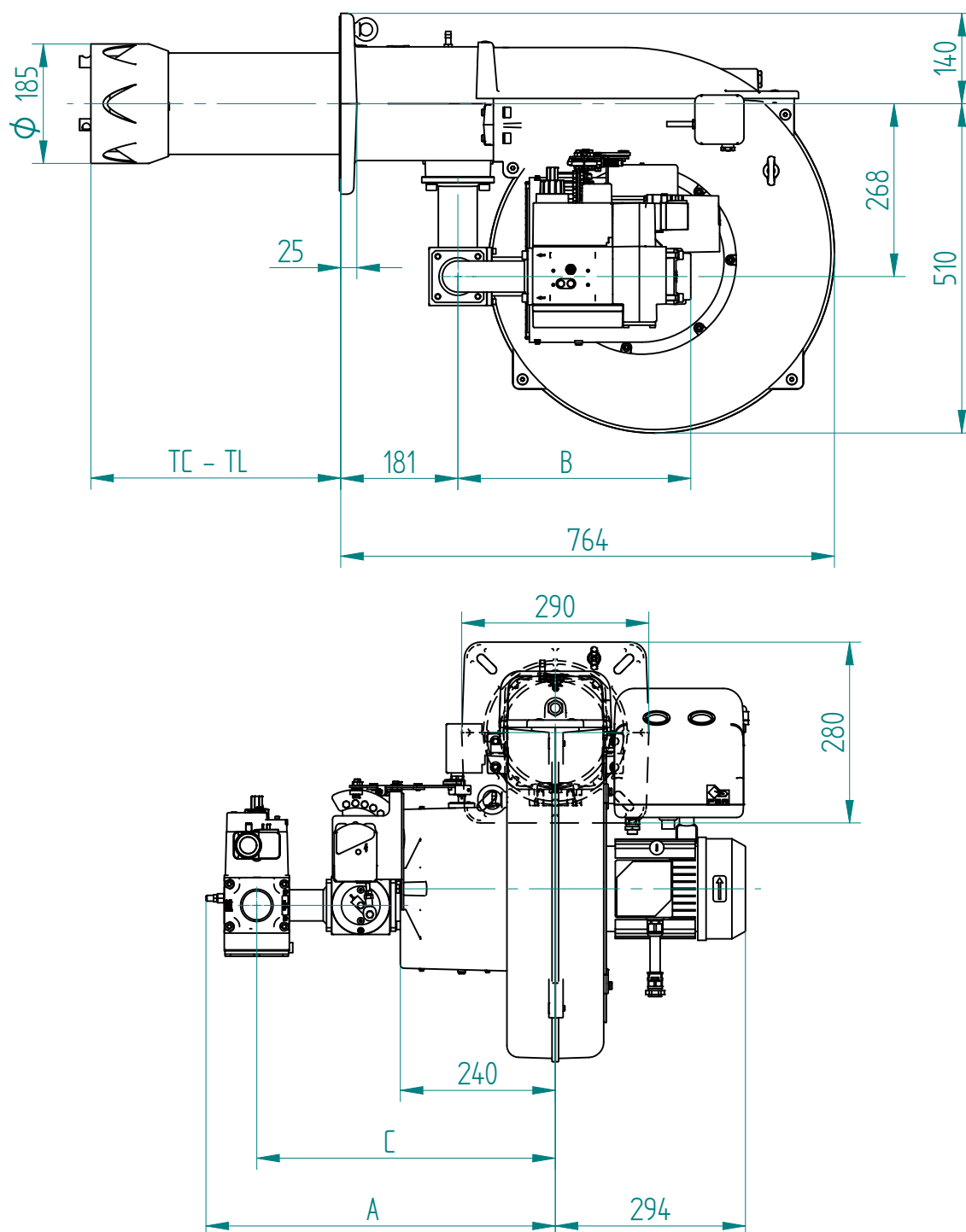
Fig. 3 Dimensions
