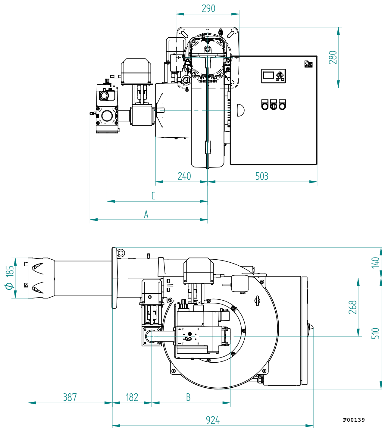
Fig. 4 Dimensions
