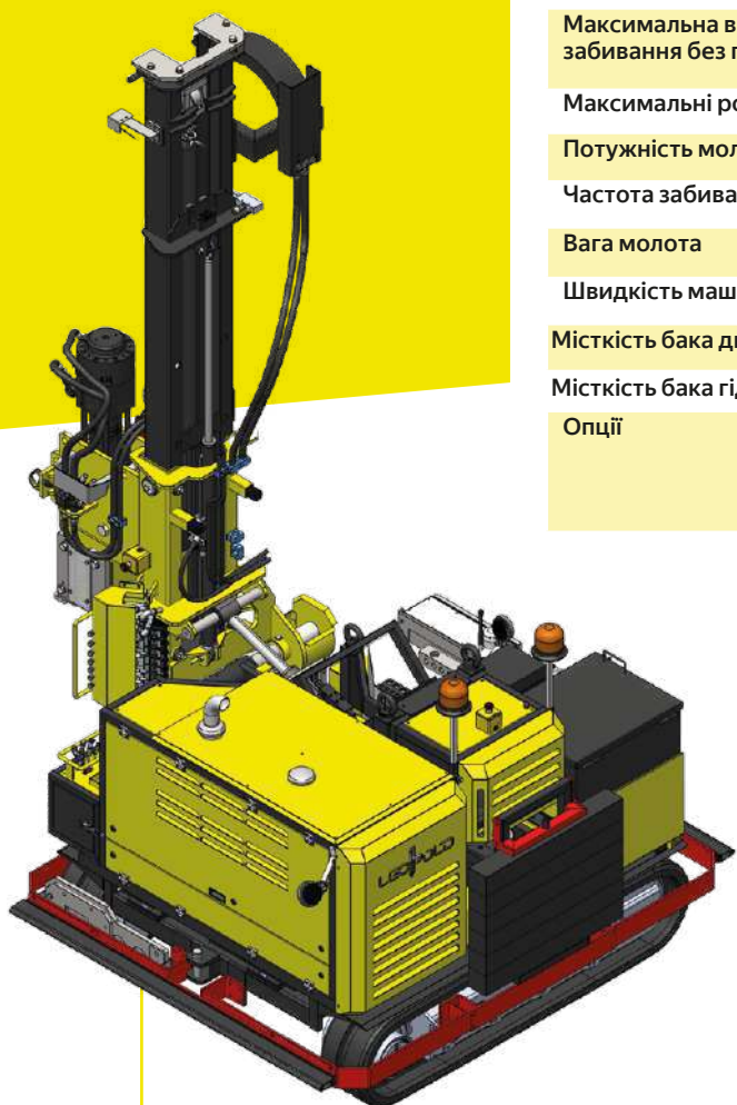
Модель: Leopold 3700 Розміри: 2400 x 2600 x h2655 mm Вага: 3825 kg Вага з баластом та ротором: 4275 kg
